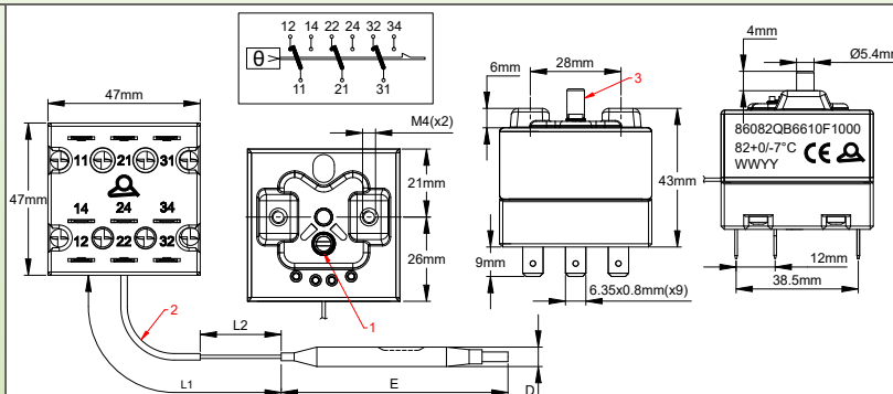
1: Versiegelter Sollwert; 2: Kapillarhülle; 3: Manuell-Reset-Taste
