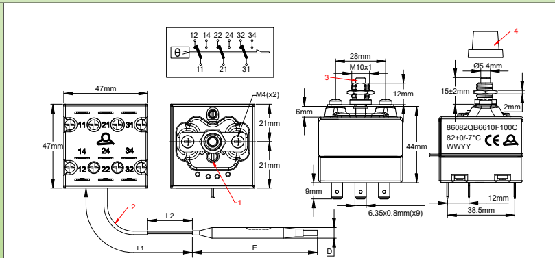
1: Versiegelter Sollwert; 2: Kapillarhülle; 3: Manuell-Reset-Taste; 4: Kappe der Manuell-Reset-Taste
